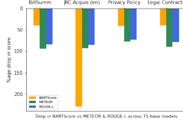
(d) BARTScore vs METEOR & ROUGE-L for T5 models
